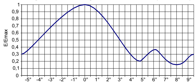
Diagrama de Elevação - Paineis 11 dBi (8,85 dBd)
