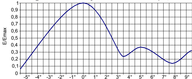
Diagrama de Elevação - Paineis 14 dBi (11,85 dBd)
