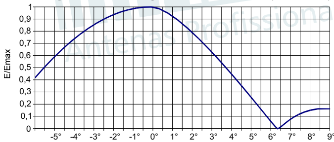
Diagrama de Elevação - Paineis 8,5 dBi (6,35 dBd)
